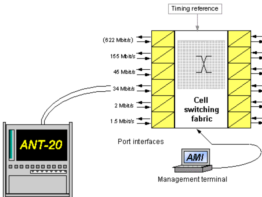
Bild E-2 Vielfältige Schnittstellenwahl beim ANT-20SE
